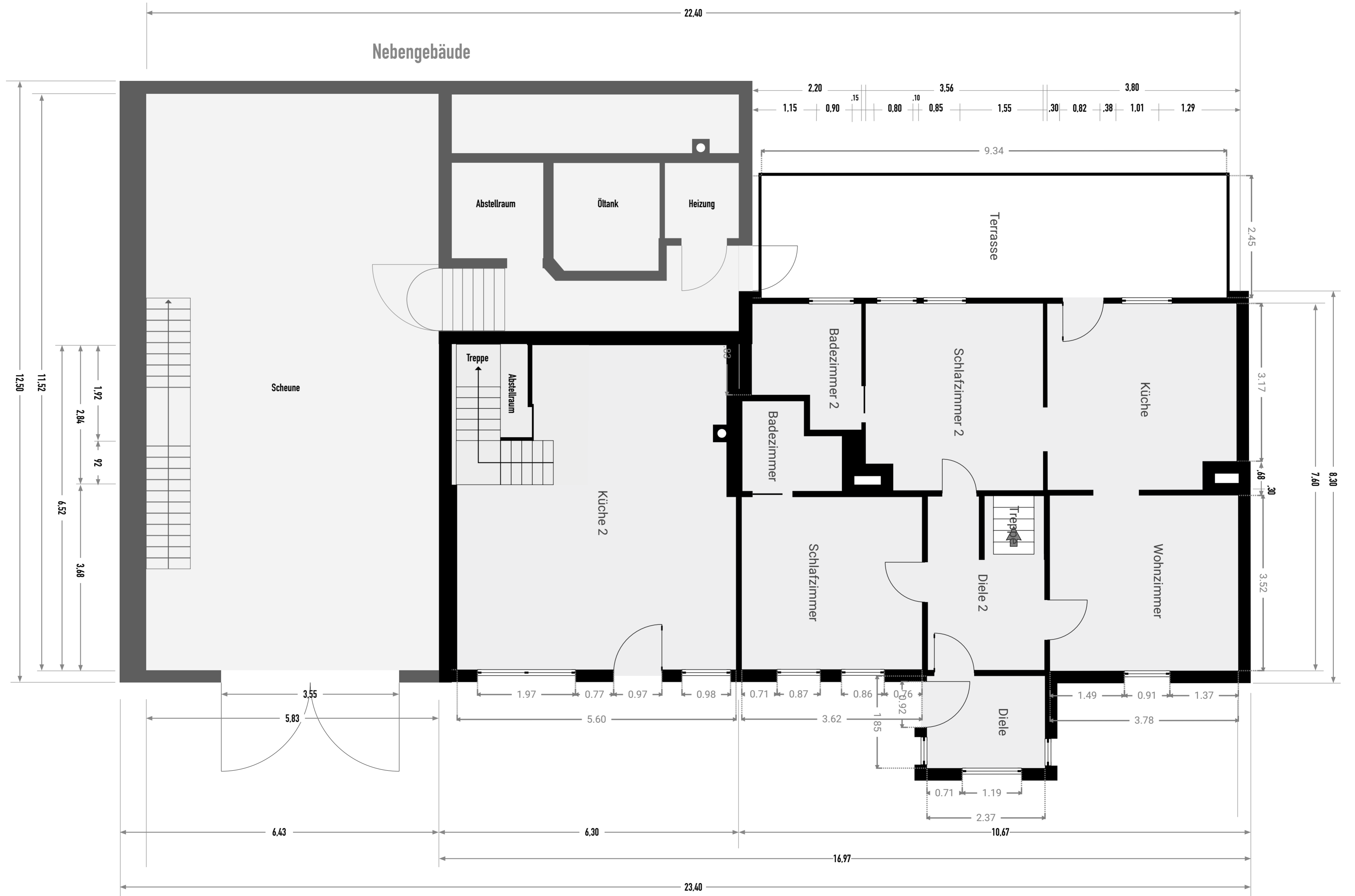
Grundriss Erdgeschoss
